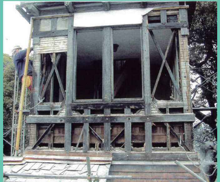
旧木内別邸 解体工事記録写真 塔屋部分
